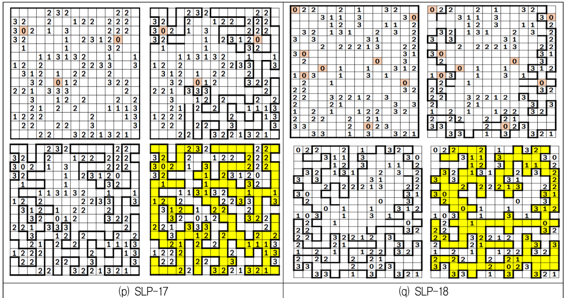
그림 7. 실험 데이터에 관한 LCA Fig. 7. LCA for experimental data
