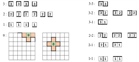
그림 3. SLP-1의 단서 선 긋기 Fig. 3. Line drawing of clue for SLP-1
