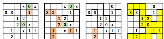
그림 5. SLP-1에 관한 LCA Fig. 5. LCA for SLP-1
