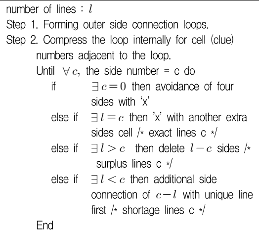
그림 4. 루프 압축 알고리즘 Fig. 4. Loop compression algorithm
