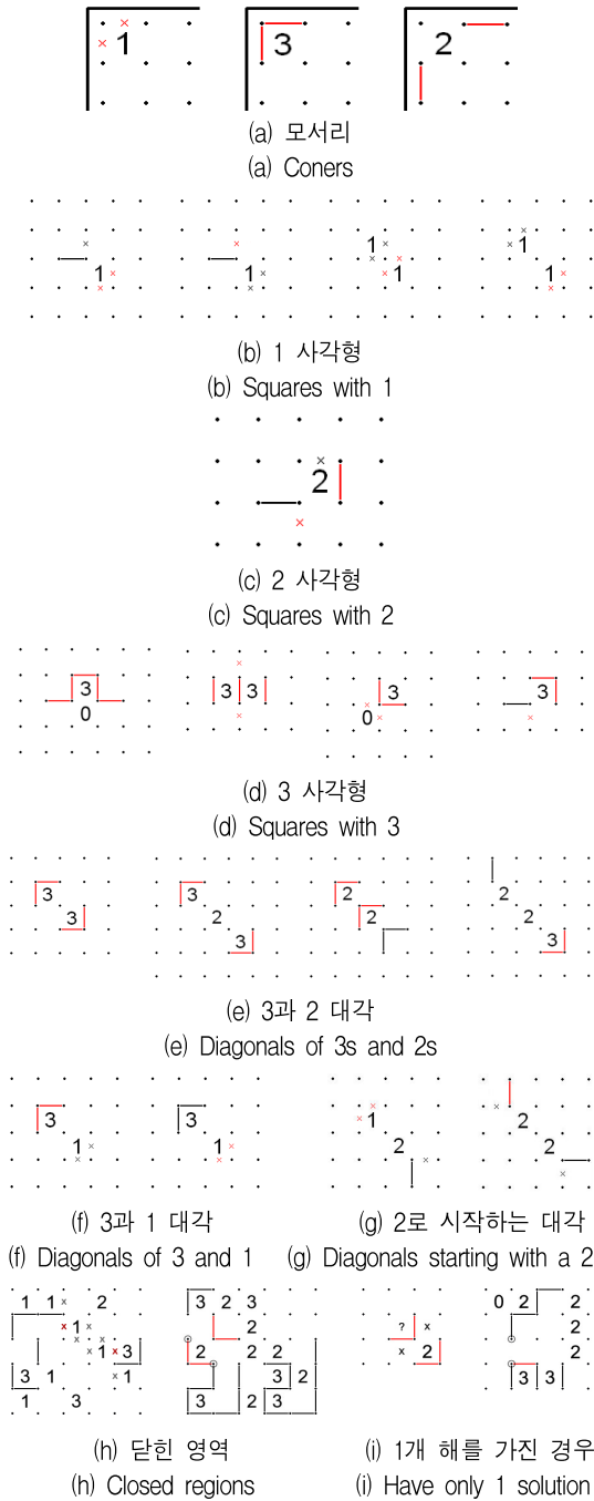
그림 2. 알려진 푸는 방법들 Fig. 2. Known solution methods
