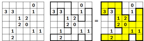
그림 1. SLP-1 슬리더링크 퍼즐 Fig. 1. Slitherlink puzzle of SLP-1
